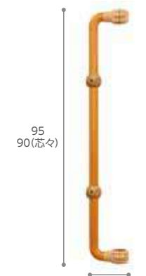
単位:cm(外寸) I型手すりロング グリップ径3.5cm
