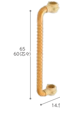
単位:cm(外寸) ウェーブ型手すりロング グリップ径3.5cm
