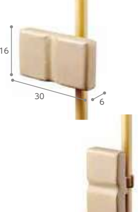
単位:cm(外寸) 膝当て手すり
