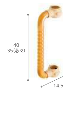
単位:cm(外寸) ウェーブ型手すり標準 グリップ径3.5cm
