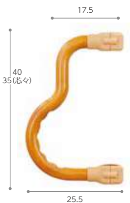
単位:cm(外寸) b型手すり グリップ径3.5cm
