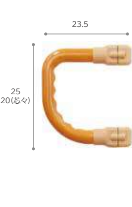
単位:cm(外寸) D型手すり グリップ径3.5cm
