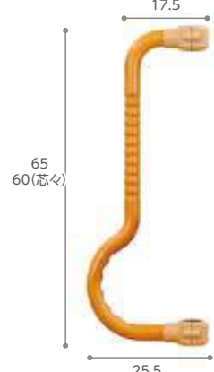
単位:cm(外寸) b型手すりロング グリップ径3.5cm
